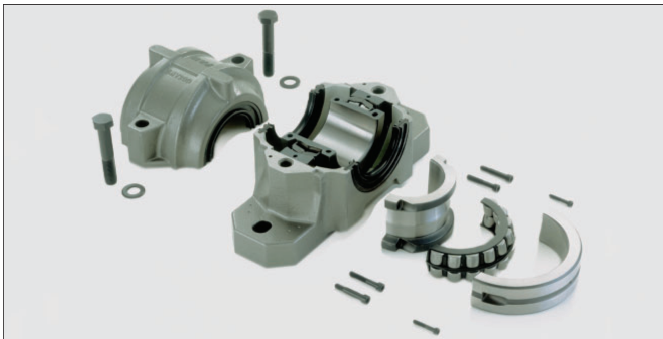
2: Helppo tarkastaa, nopea ja yksinkertainen asentaa - jaetun pallomaisen rullalaakerin asennus SNV-pesään
