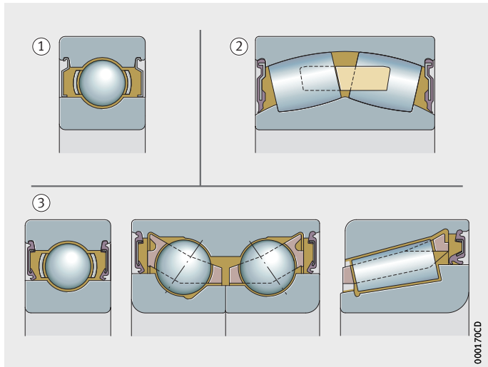
Kuva 7 Tiivistetyt laakerit
