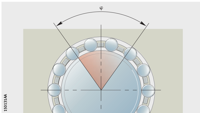
Kuva 5 Kääntökulma
