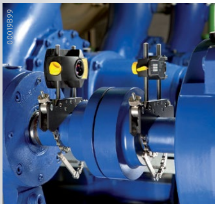
Lähetin ja vastaanotin asennettuna
